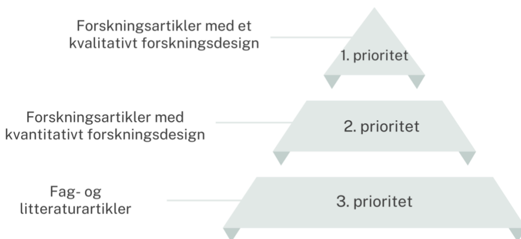
Figur 2: Litteraturhierarkiet
