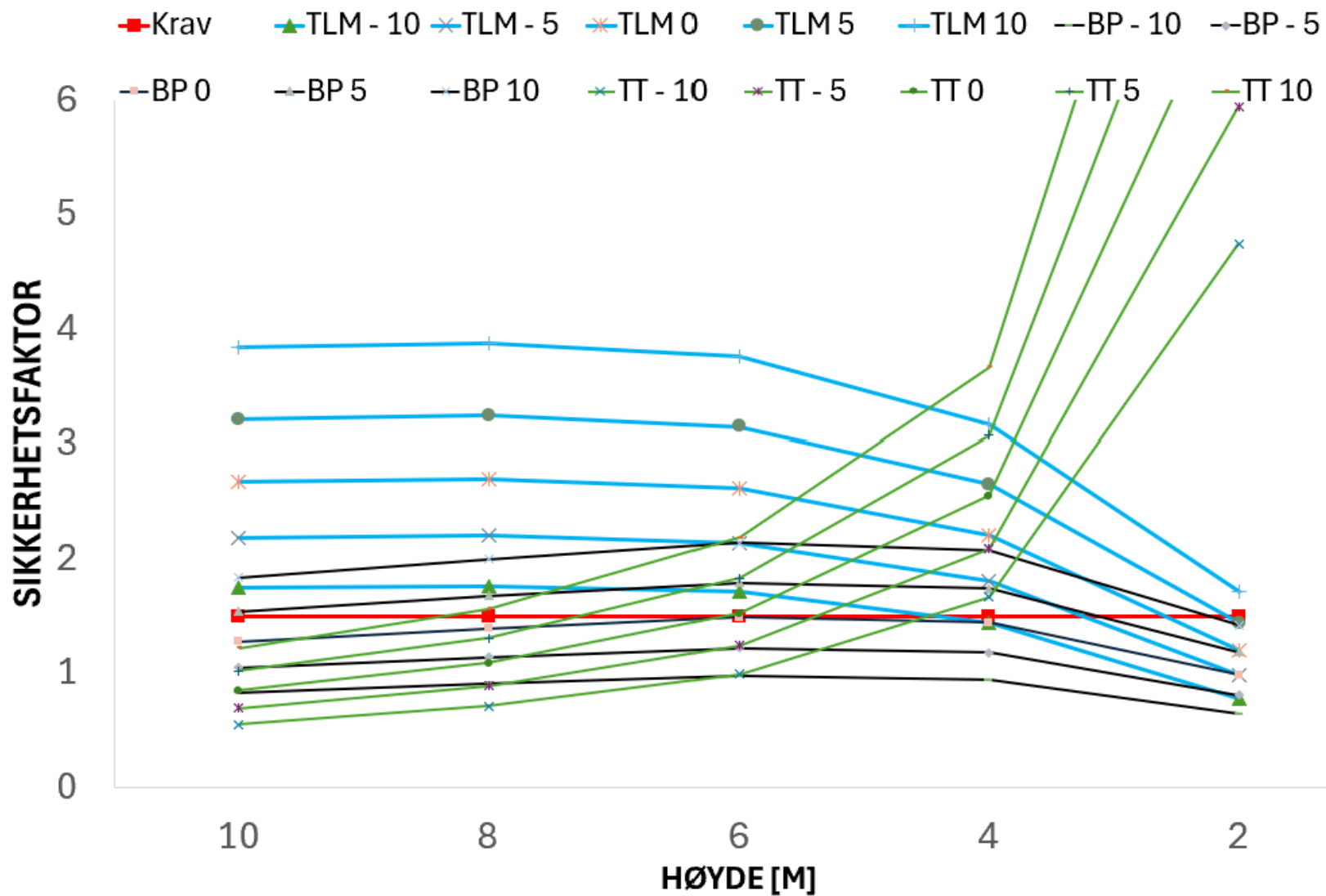
Figur 3 Glidestabilitet samlet, HRV b[4m] islast[100kN/m]
