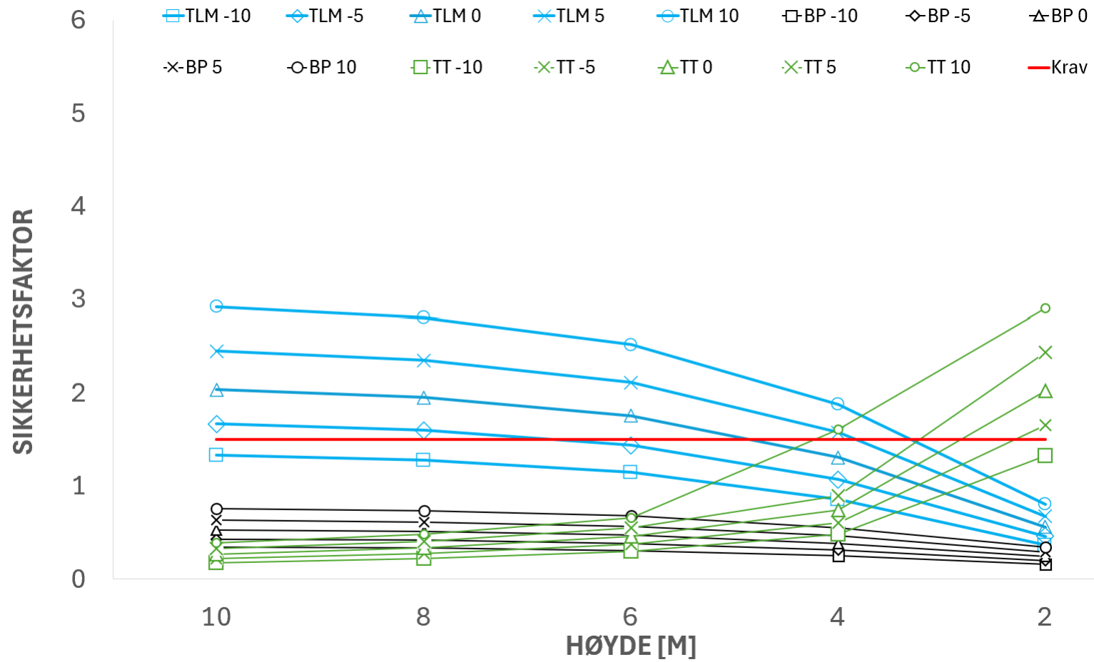
Figur 1 Glidestabilitet samlet, HRV b[1m] islast[100kN/m]
