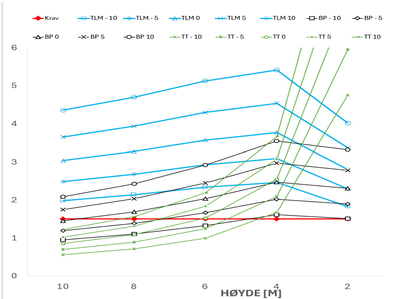
Figur 6 Glidestabilitet samlet, HRV b[4m] islast[40kN/m]
