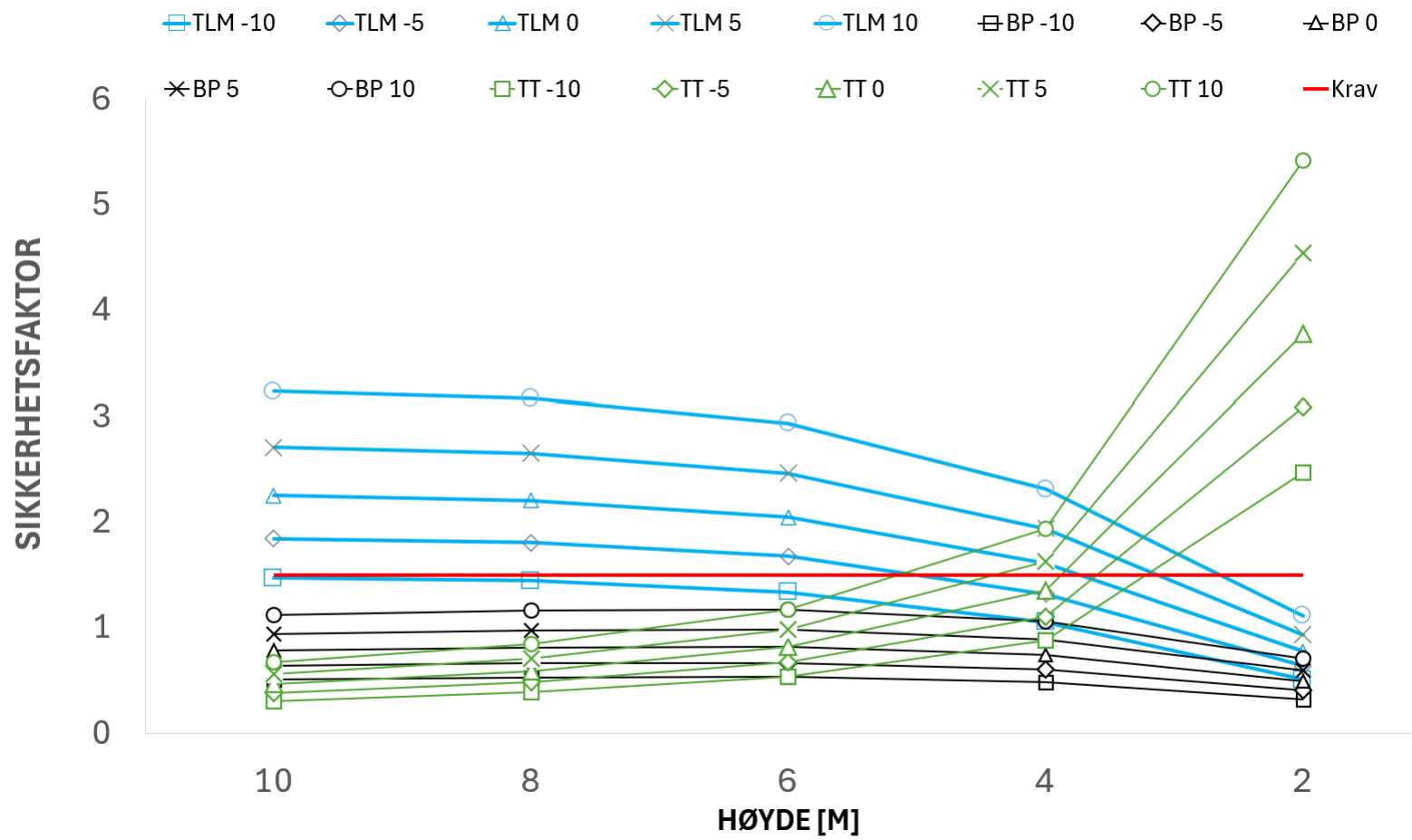
Figur 2 Glidestabilitet samlet, HRV b[2m] islast[100kN/m]
