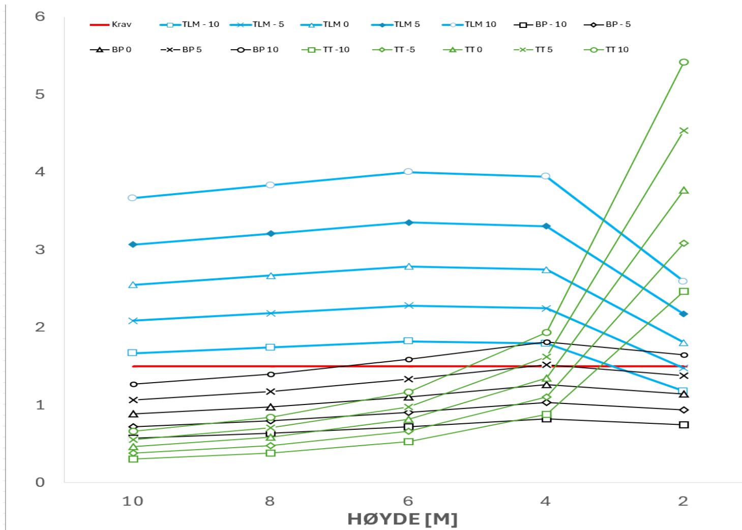
Figur 5 Glidestabilitet samlet, HRV b[2m] islast[40kN/m]
