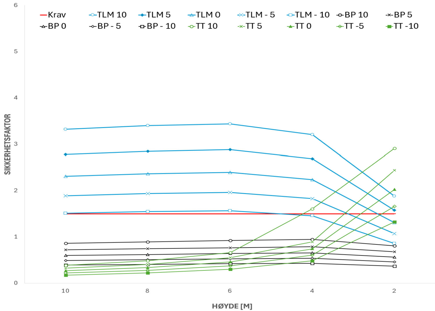
Figur 4 Glidestabilitet samlet, HRV b[1m] islast[40kN/m]
