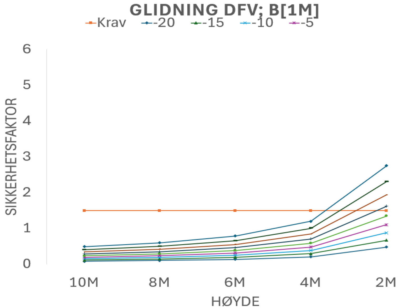
Figur 4 TT, Glidning DFV b[2m] islast[0kN/m]
