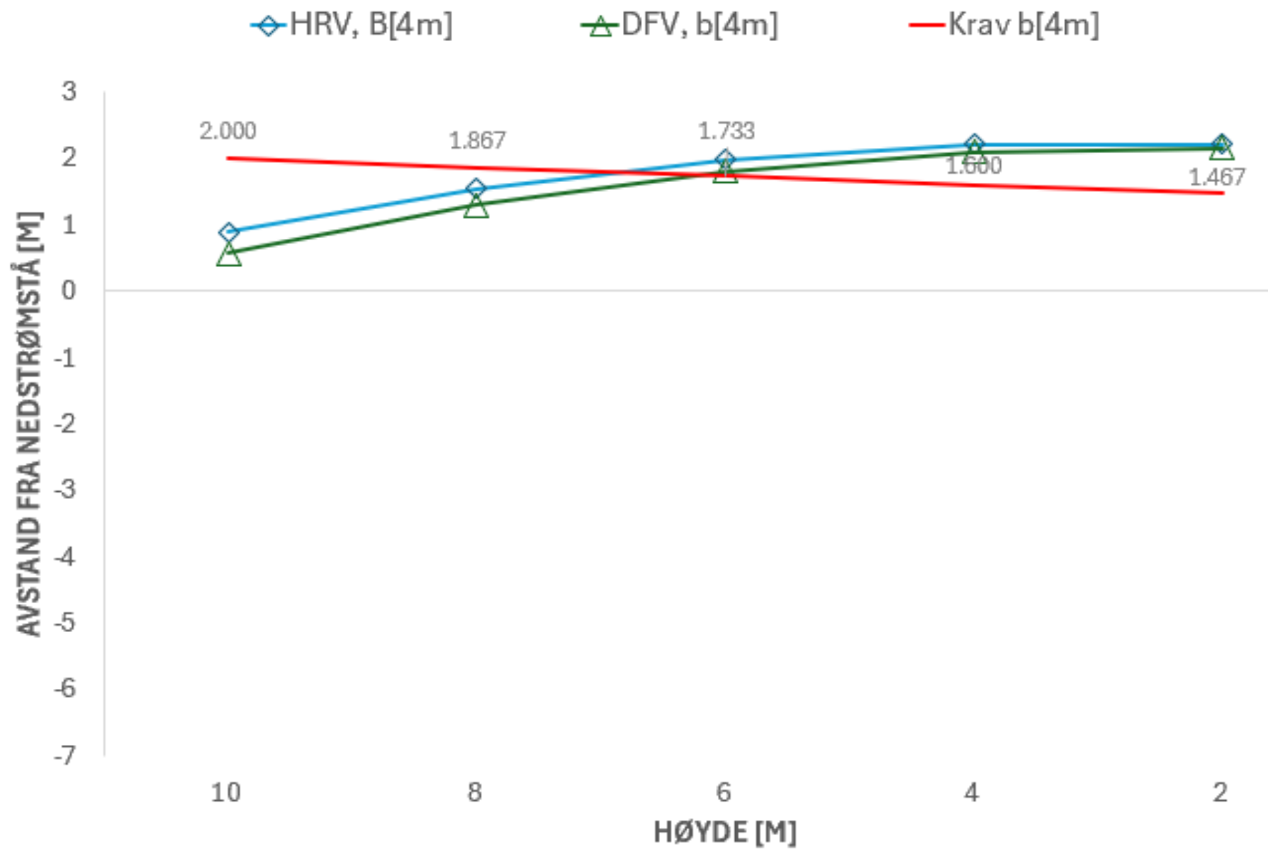
Figur 9 TT, Veltestabilitet b[4m]
