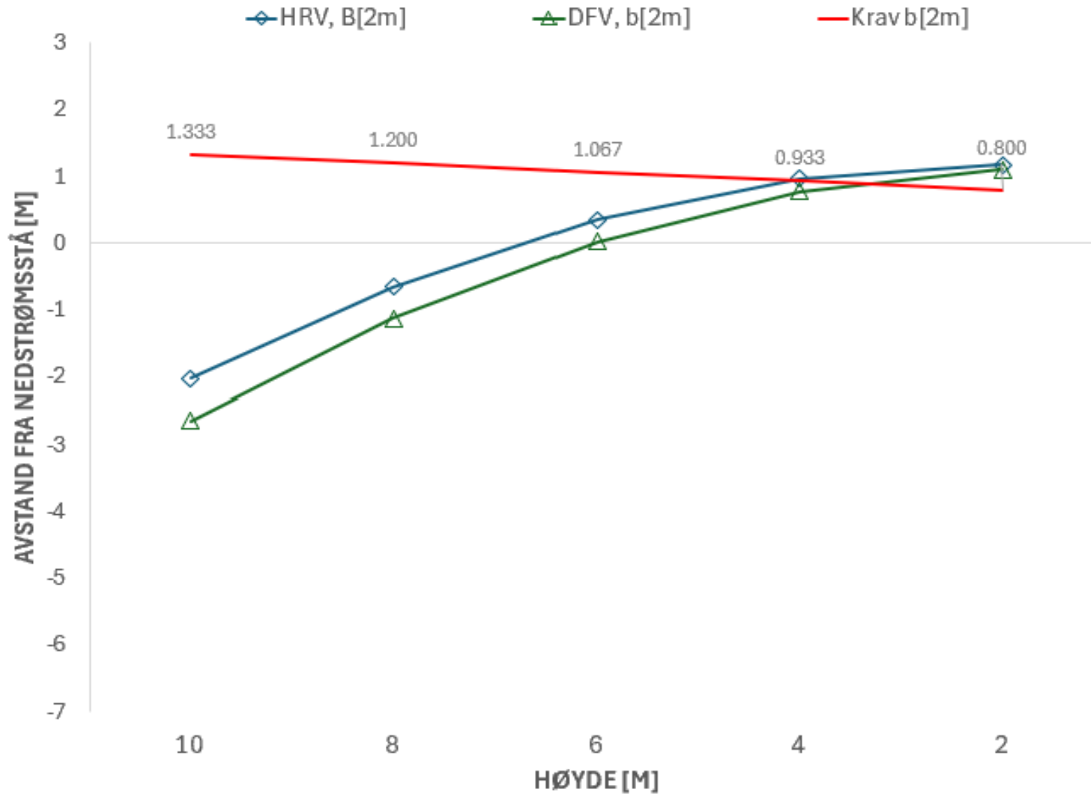
Figur 8 TT, Veltestabilitet b[2m]
