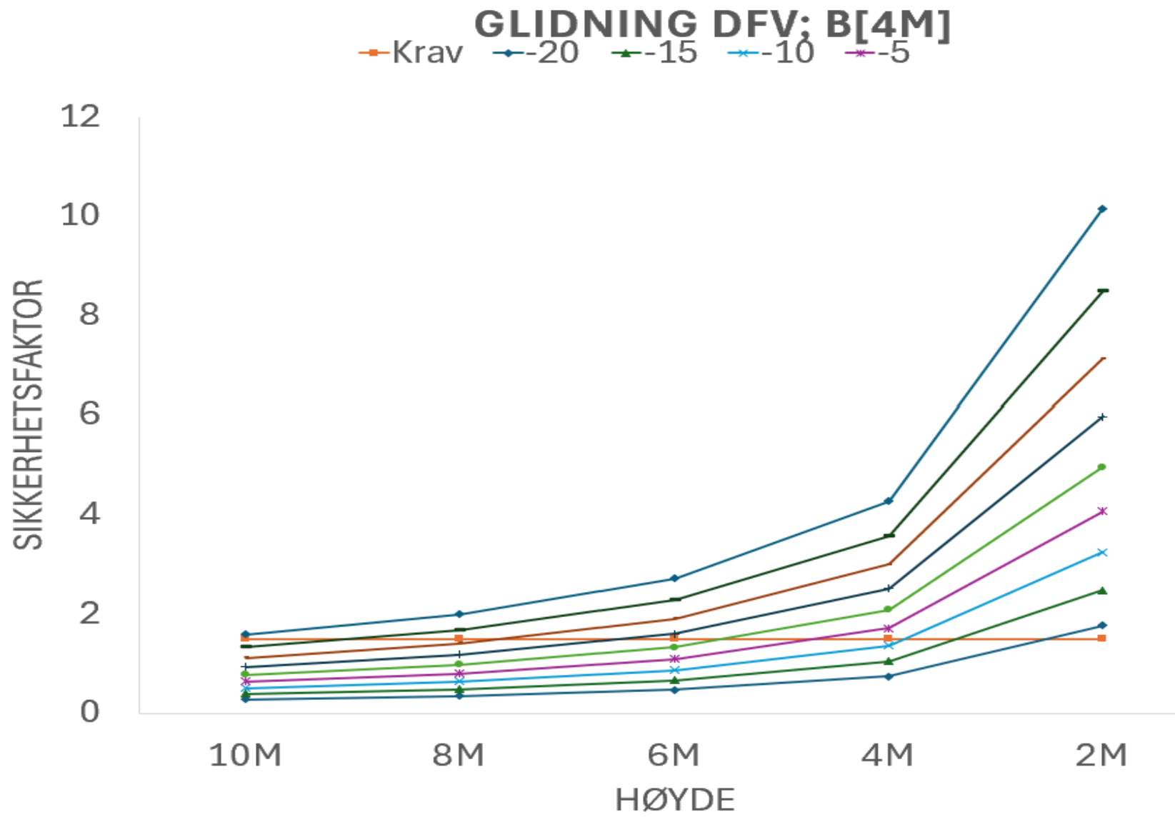
Figur 6 TT, Glidning DFV b[4m] islast[0kN/m]
