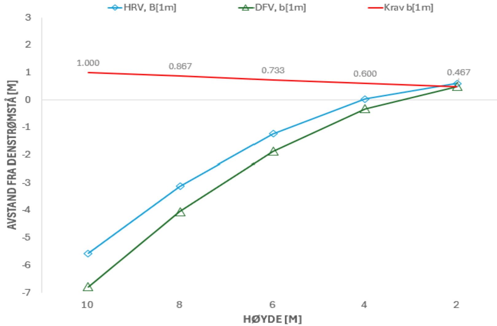
Figur 7 TT, Veltestabilitet b[1m]
