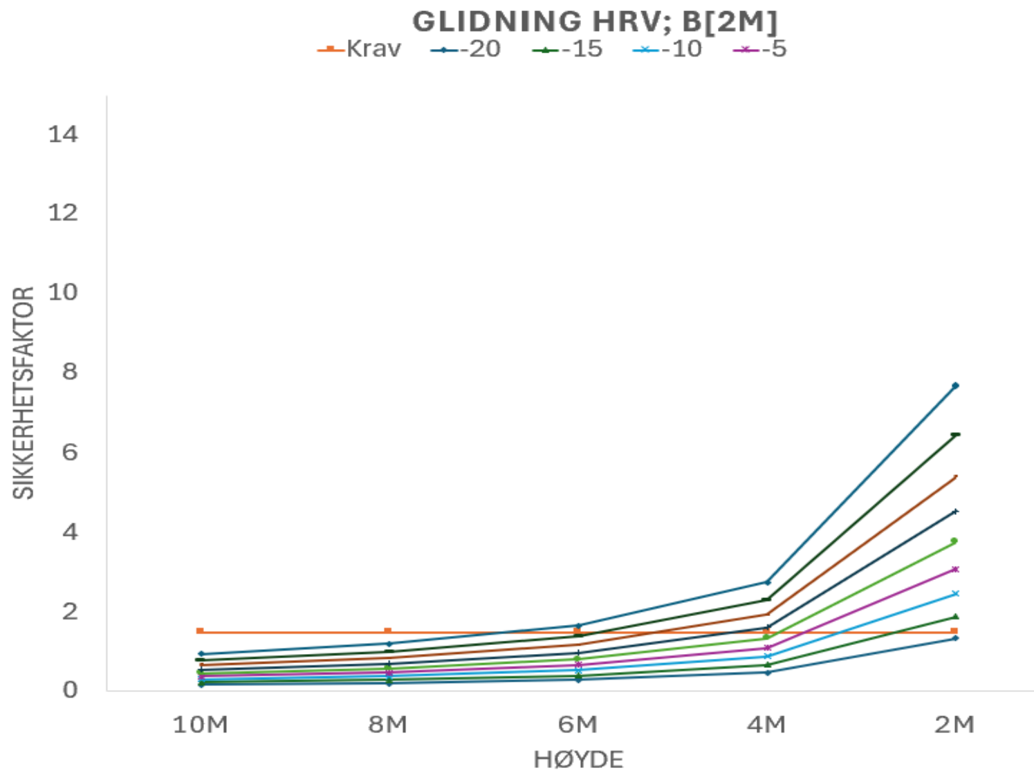
Figur 2 TT, Glidning HRV [2m] islast[0kN/m]
