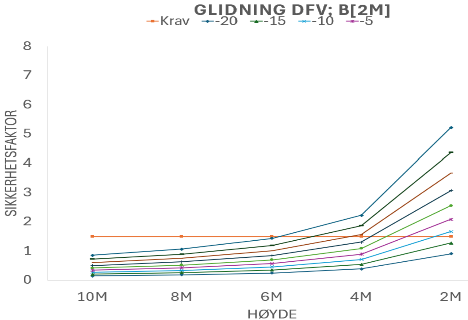
Figur 5 TT, Glidning DFV b[2m] islast[0kN/m]
