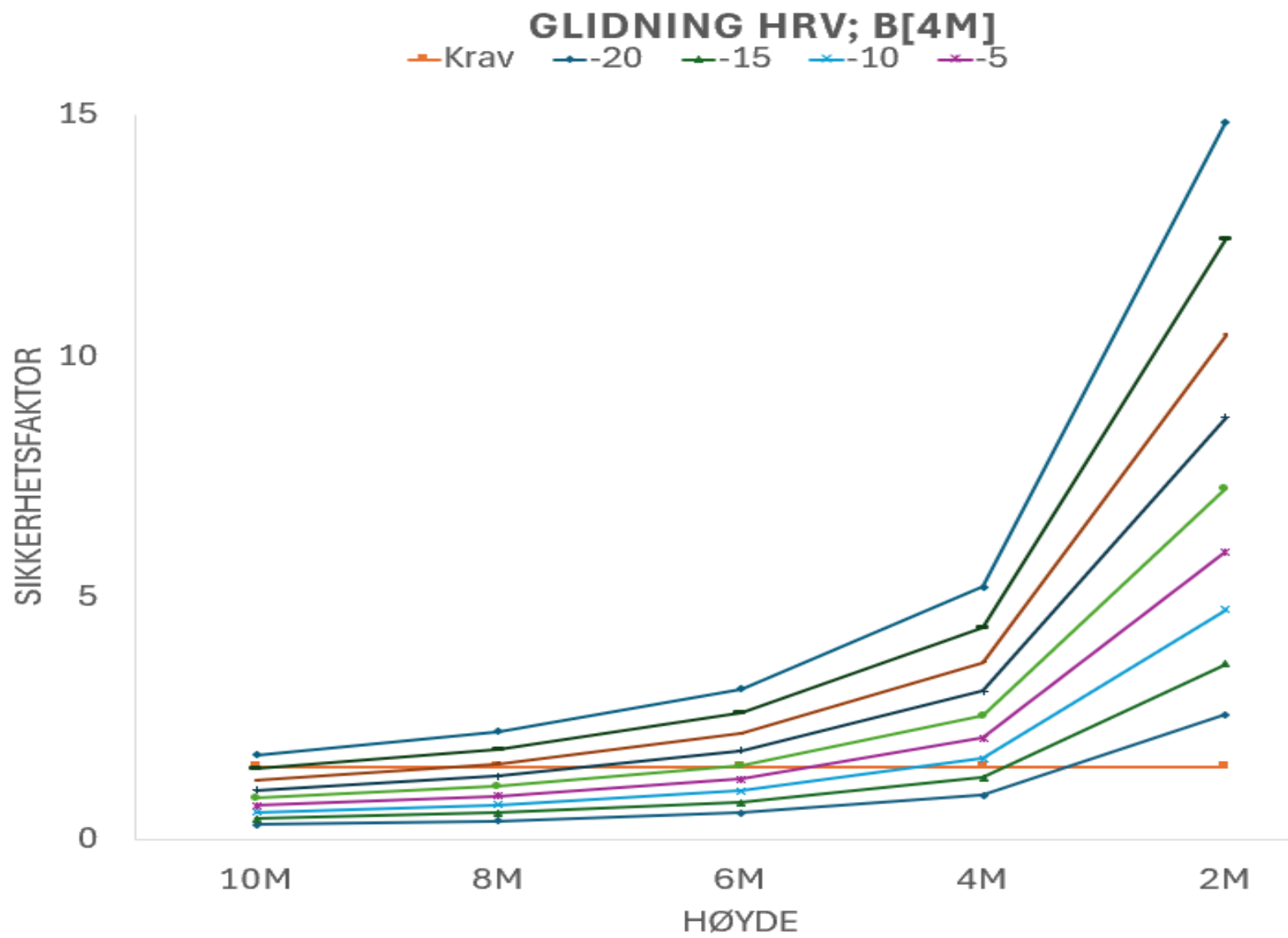
Figur 3 TT, Glidning DFV b[1m] islast[0kN/m]
