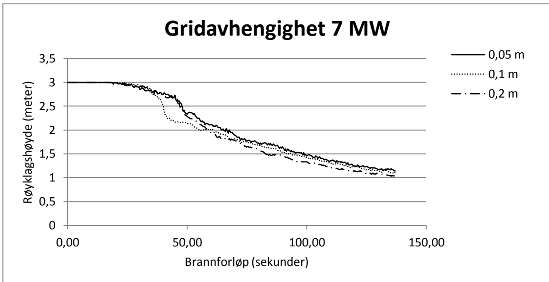
Figur 31 - Løsning konvergerer ved branneffekt 7 MW.
