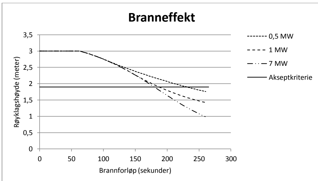
Figur 28 – Branneffekt
