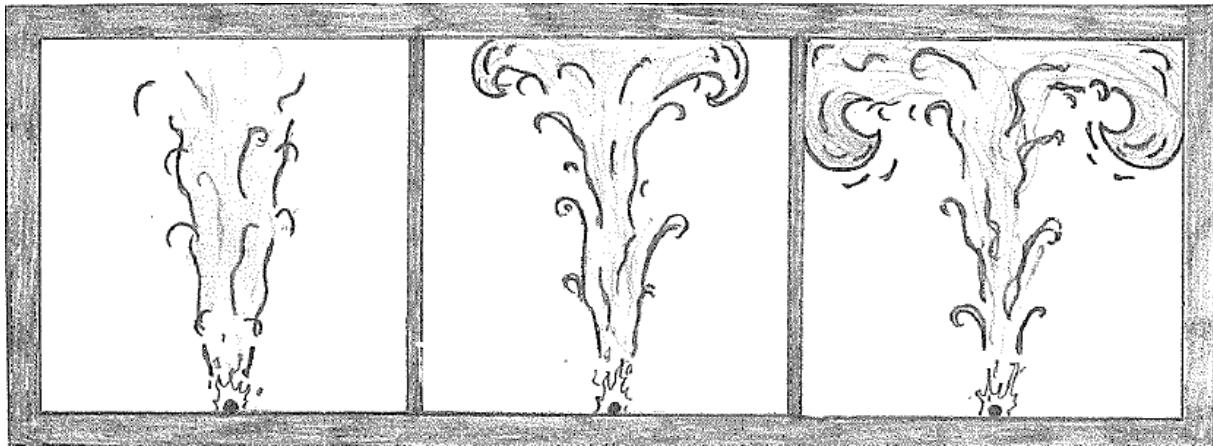
Figur 4 – Dannelse av røyklag. Bildet til venstre: røyksøyle er dannet. Bildet i midten: Røyksøyle treffer taket og danner en takjet. Bildet til høyre: Røyk avbøyes ved veggene.
