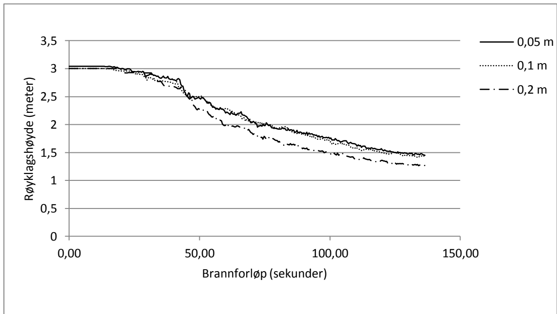
Figur 14 - Løsning konvergerer ved maksimal branneffekt 0,5 MW for cellestørrelsene 0,1 og 0,05 meter.
