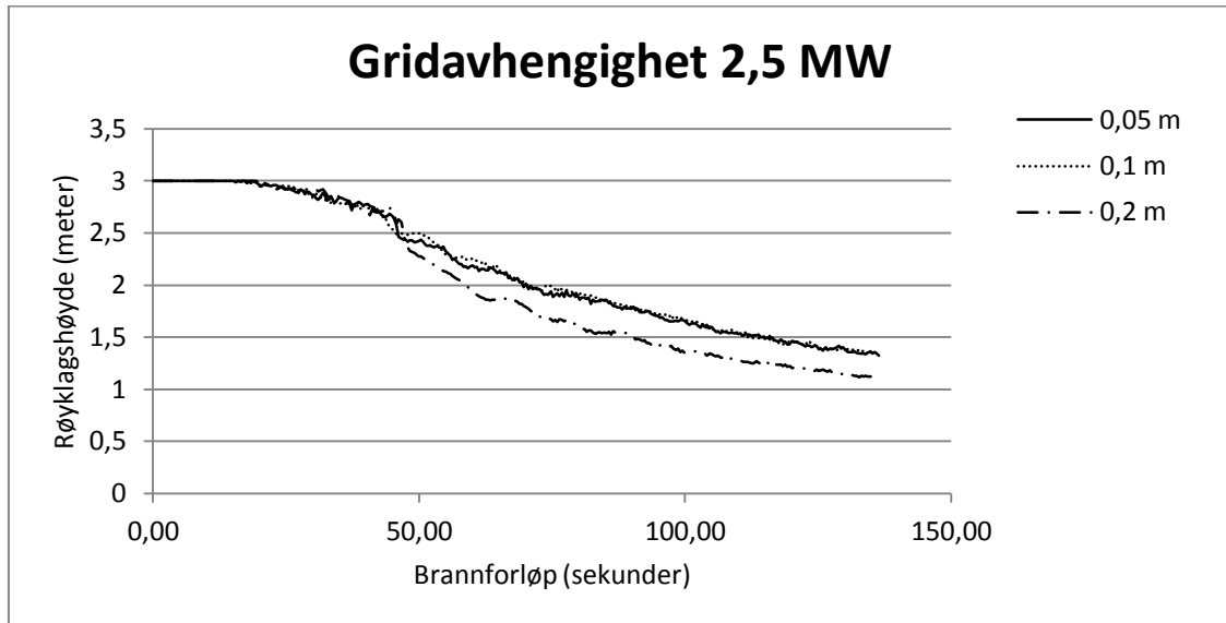
Figur 30 - Løsning konvergerer ved branneffekt 2,5 MW for cellestørrelsene 0,1 og 0,05 meter
