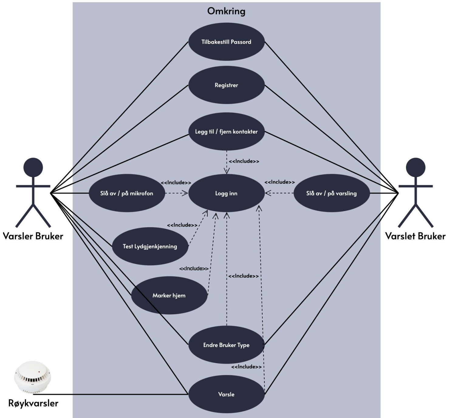
Figur 1: Brukstilfellediagram
